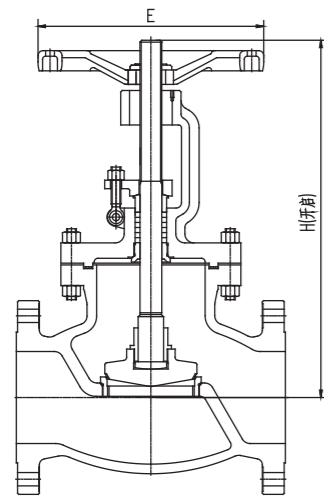
Yoke 带支架 PN63, DN≥200 PN100, DN≥200
